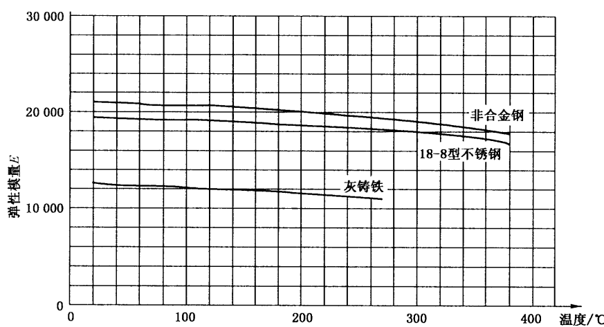
图 B.1 作为温度函数的弹性模量 E 的变化
