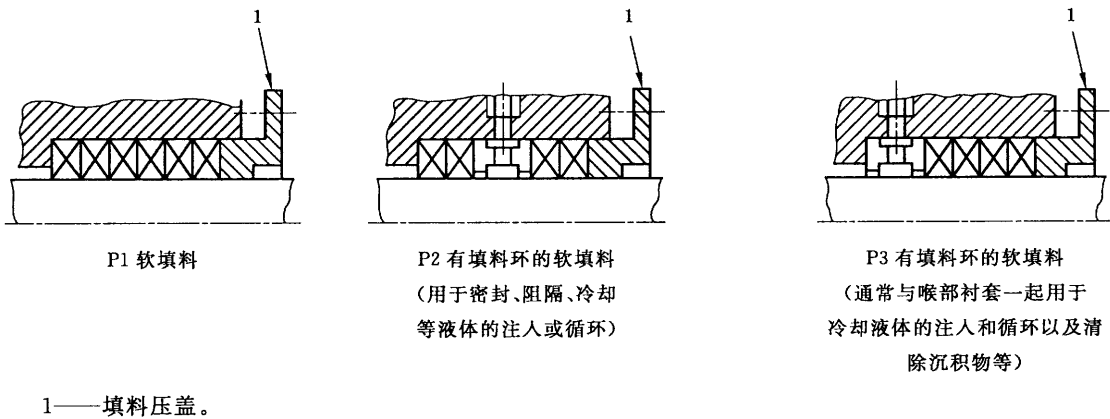
图 E.1 软填料密封的示例
